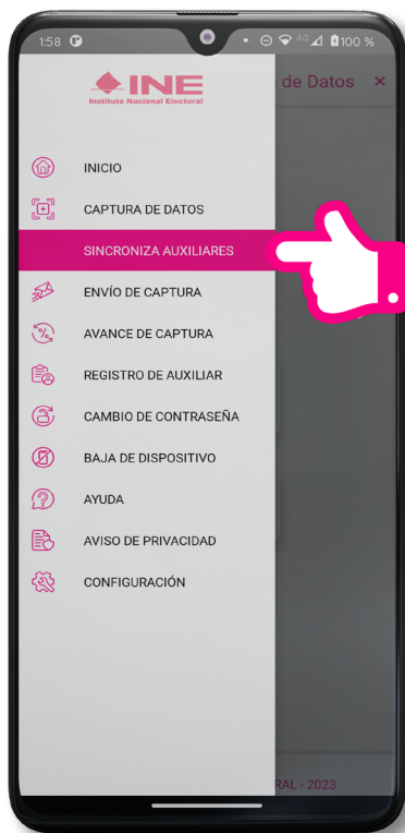
Figura 78. Sincronización Auxiliares.
