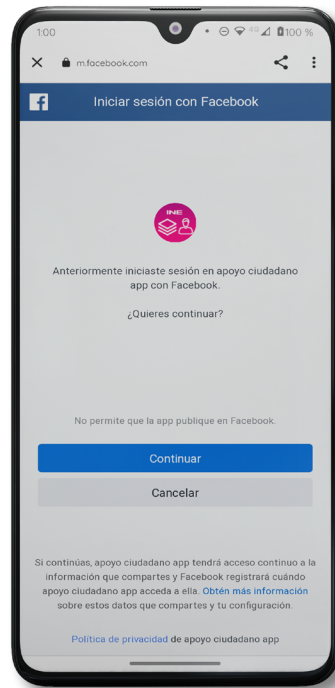
Figura 69. Autenticación Facebook.
