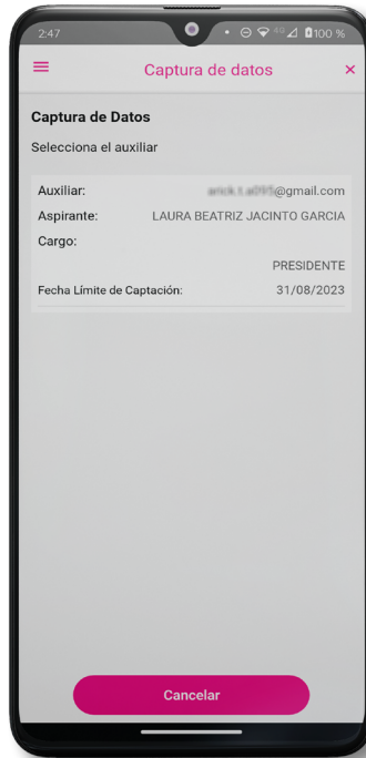
Figura 38. Auxiliar registrado.
