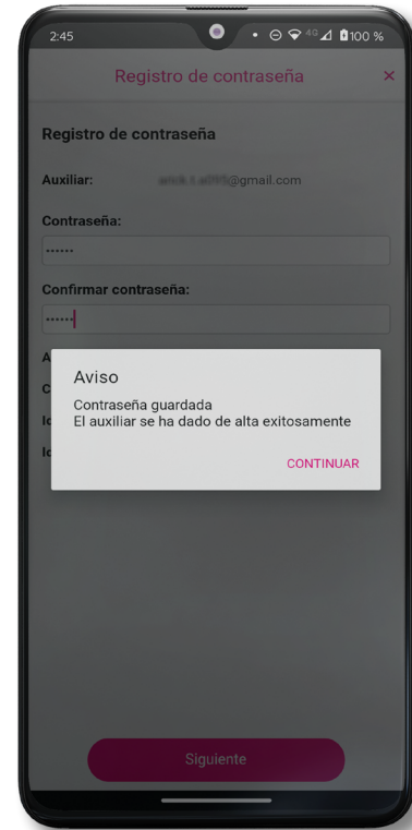
Figura 34. Contraseña guardada.
